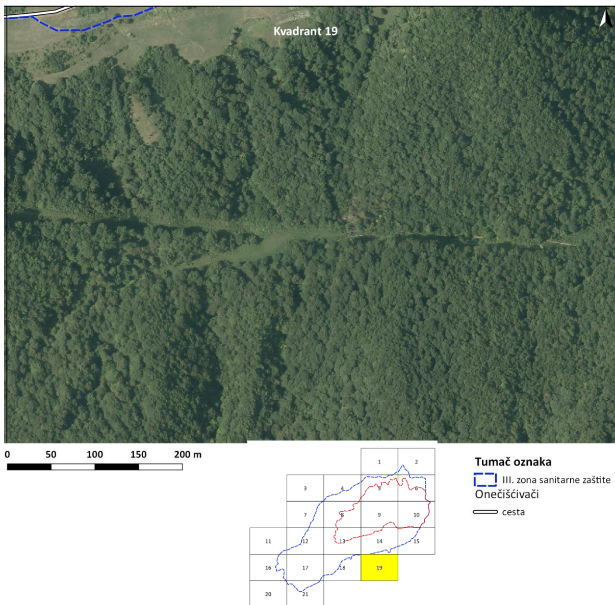
Grafički prikaz 4-20: Kvadrant 19 – prikaz onečišćivača
